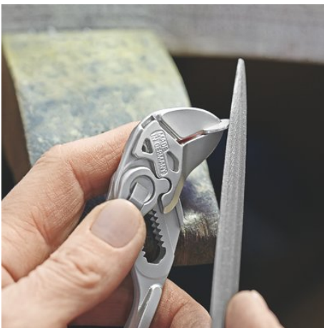
der Mini-Zangenschlüssel für feinmechanische Arbeiten
